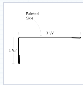
1.5"x3.5" L-Trim (2-Hems)
