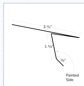
S.S. Drip Edge
