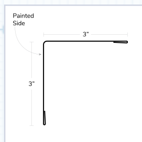
3"x3" L-Trim (2-Hems)
